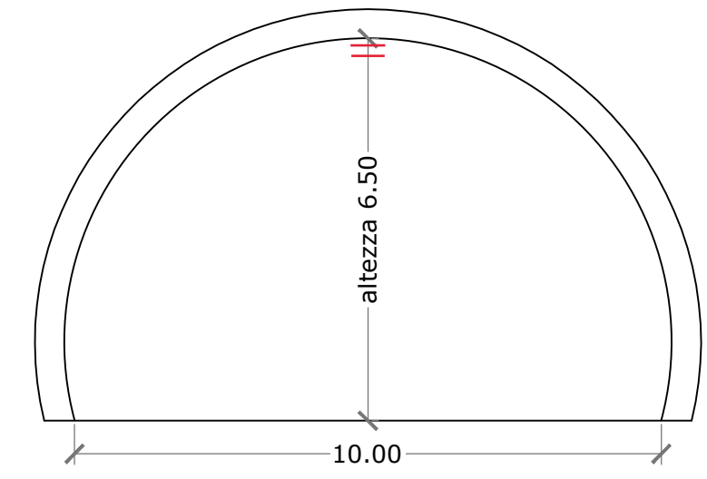
SEZIONE TIPO GALLERIA
